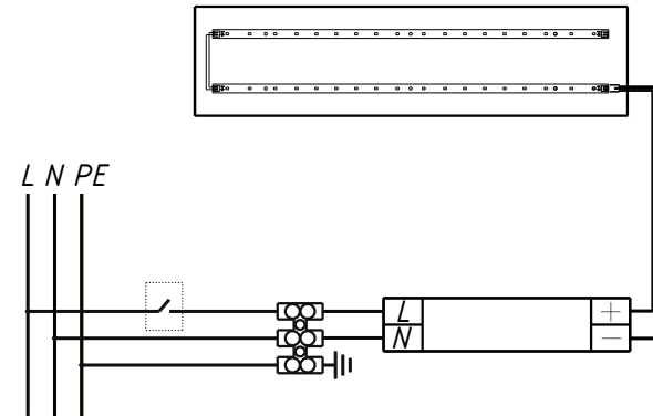
Рисунок 1 - Схема подключения светильников
